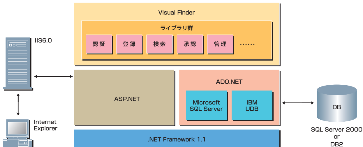
図1：Visual Finder 4.0の内部構造
