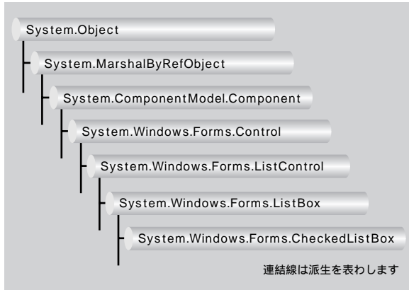
図1: CheckedListBox階層図
